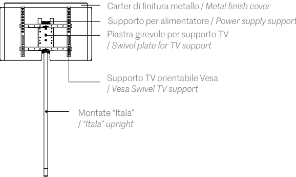
ROTAZIONE SUPPORTO TV / TV SUPPORT ROTATION
