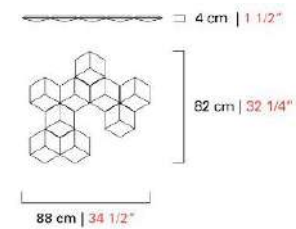
7253W/9 L880*E40*H820mm
