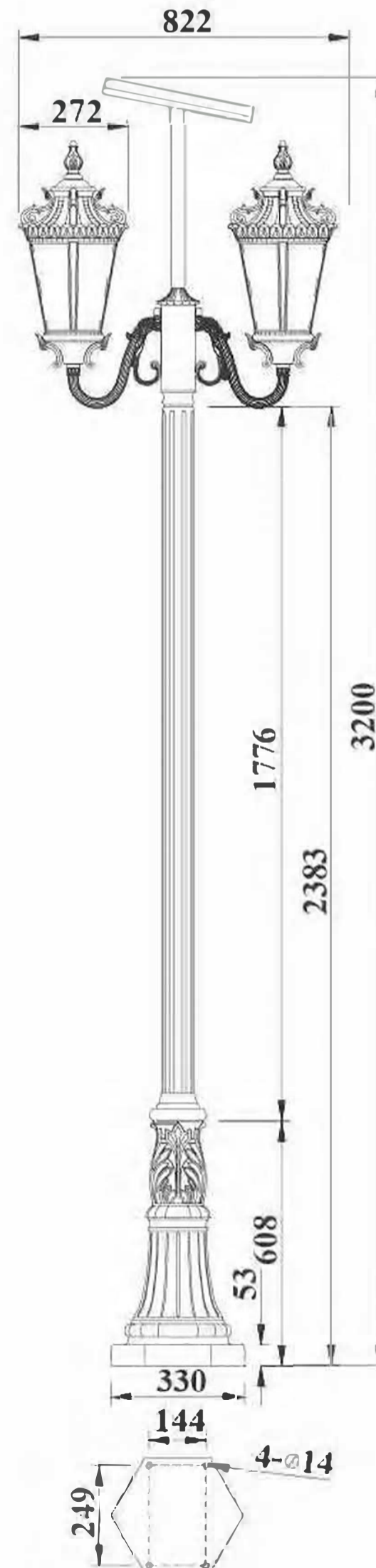
E-3239-2MA (58#) (Unit: mm)
