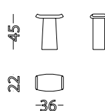
mod. 9090002 Sgabello
