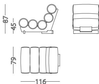
mod. 1480001 Poltrona
