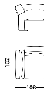
mod. 6500015 Pouf
