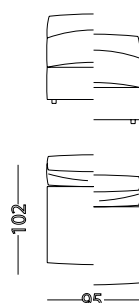
mod. 650006 Elemento 95
