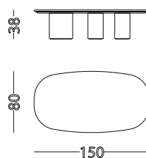
mod. 9010001
