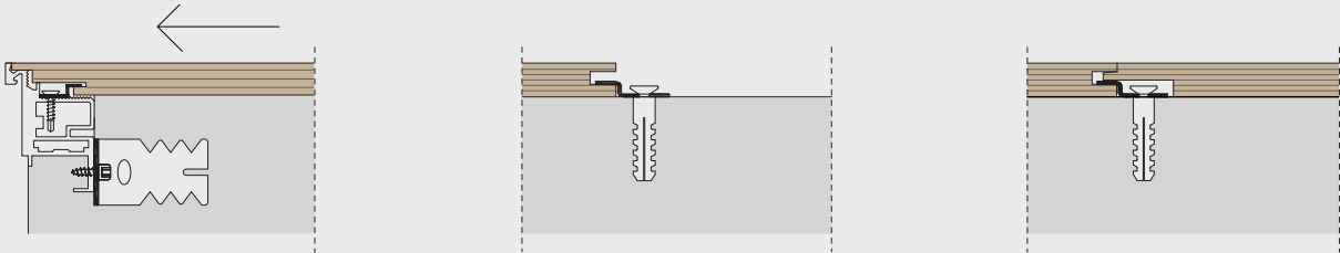
Installazione pannello iniziale Installation of the starting panel
