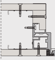
Cartongesso Plasterboard
