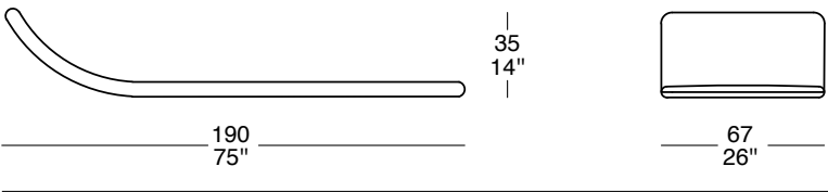
CHAISE LONGUE CON CUSCINO CHAISE LONGUE WITH CUSHION
