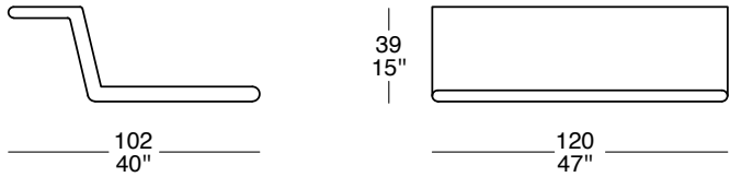
EL. SINGOLO CON CUSCINO SEDUTA/SCHIENALE SINGLE EL. W/ SINGLE SEAT/BACK CUSHION
