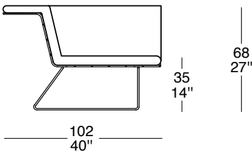
ANGOLO C/CUSC.SEDUTA/SCHIENALE C/MENSOLA ANGOLO W/SEAT/BACK CUSH/SHELF
