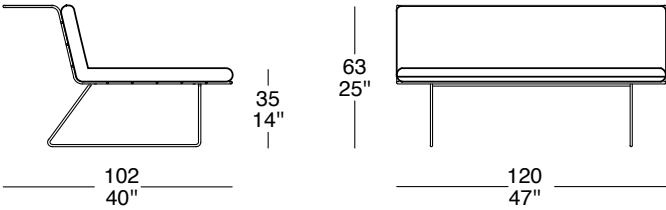
EL. SINGOLO CON CUSCINO SEDUTA/SCHIENALE SINGLE EL. W/ SINGLE SEAT/BACK CUSHION
