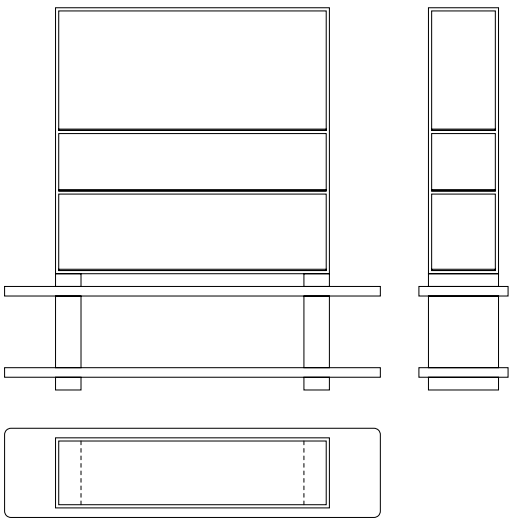
bookshelf n°1 — GSMA731 cm 236 x 56 | h. cm 240
