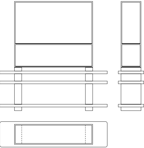
bookshelf n°2 — GSMA831 cm 236 x 56 | h. cm 240
