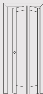
Apertura a libro. Bi-fold door.
