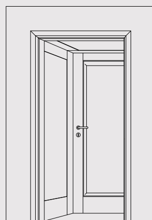
Telaio intelaiato rettangolare. Special frame - rectangular.
