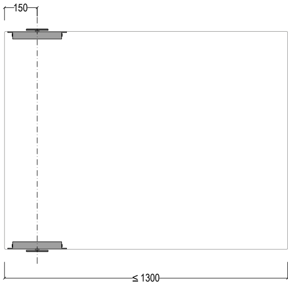
Cerniera porta a bilico e posizionamento sull'anta _Pivot door's hinge and positioning on the door
