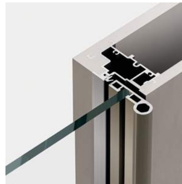
Porta a battente 180 su stipite Plain
