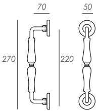
Pull Handle Manillón
