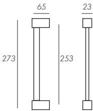
Pull Handle Manillón
