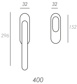
Lifter Pull Handle Manillón Elevador
