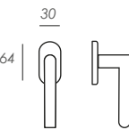
Window Handle Grisán
