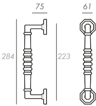
Pull Handle Manillón
