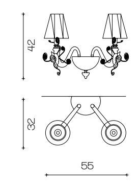
Art. 1631/A2 L 55 cm H 42 cm Sp 32 cm PØ 16 cm 2 x E14 x 40W
