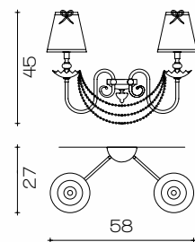
Art. 1794/A2 L 58 cm H 45 cm Sp 27 cm Pø 16 cm 2 x E14 x 40W
