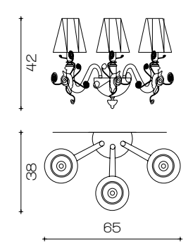
Art. 1631/A3 L 65 cm H 42 cm Sp 38 cm PØ 16 cm 3 x E14 x 40W
