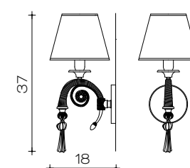
Art. 1162/A P Ø 18 cm H 37 cm Sp 18 cm 1 x E14 x 40W
