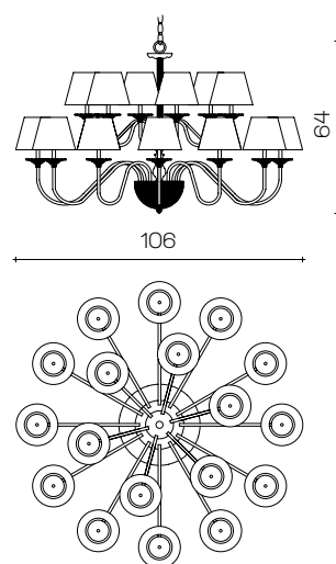
Art. 1460/CH18 ø 106 cm H 64 cm Pø 16 cm 18 x E14 x 40W
