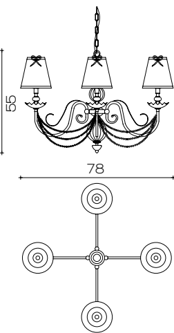
Art. 1794/CH4 Ø 78 cm H 55 cm Pø 16 cm 4 x E14 x 40W
