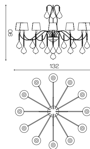
Art. 1742/CH12/KR/V1 ø 132 cm H 90 cm Pø 14 cm 12 x E14 x 25W
