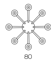
Art. 1761/CH8 Ø 80 cm H 90 cm PØ 16 cm 8 x E14 x 40W
