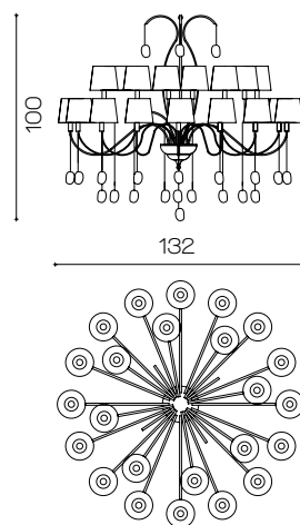
Art. 1710/CH24/OV ø 132 cm H 100 cm Pø 14 cm 24 x E14 x 25W
