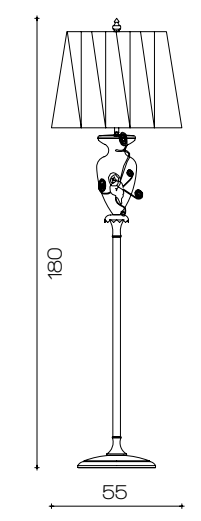
Art. 1631/FL H 180 cm PØ 55 cm 2 x E27 x 60W
