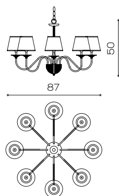
Art. 1460/CH8 ø 87 cm H 50 cm Pø 16 cm 8 x E14 x 40W
