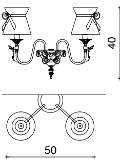
Art. 1850/A2 L 50 cm H 40 cm Sp 28 cm 2 x E14 x 40W
