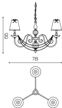
Art. 1794/CH3 Ø 78 cm H 55 cm Pø 16 cm 3 x E14 x 40W
