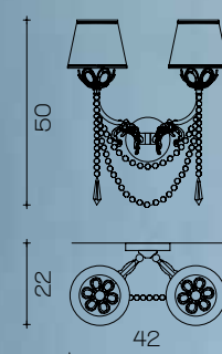
Art. 1744/A2/ORO24K ø 42 cm H 50 cm Pø 16 cm Sp 22 cm 2 x E14 x 40W
