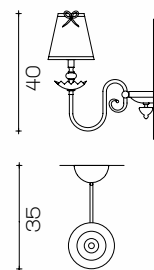
Art. 1794/A1 H 40 cm Sp 35 cm Pø 16 cm 1 x E14 x 40W
