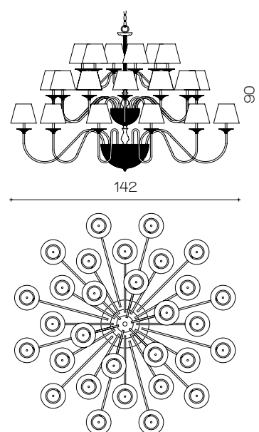
Art. 1460/CH30 ø 142 cm H 90 cm Pø 16 cm 30 x E14 x 40W
