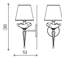
Art. 777/A Pø 16 cm H 38 cm Sp 19 cm 1 x E14 x 40W
