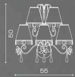
Art. 1627/A5 ø 55 cm H 50 cm Sp 15 cm Pø 14 cm 5 x E14 x 40W
