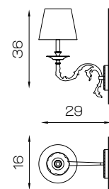
Art. 1986/A1 ø 16 cm H 36 cm Pø 16 cm Sp 29 cm 1 x E14 x 40W
