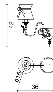
Art. 1850/A1 H 42 cm PØ 16 cm Sp 36 cm 1 x E14 x 40W
