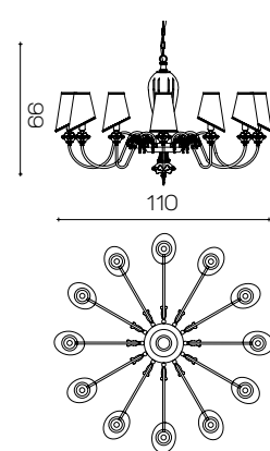
Art. 1774/CH12 ø 110 cm H 66 cm Pø 14 cm 12 x E14 x 40W
