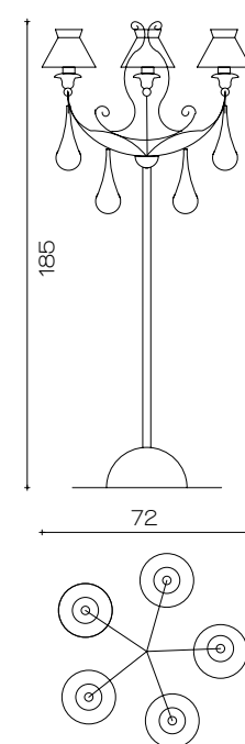
Art. 1823/FL ø 72 cm H 180 cm Pø 20 cm 5 x E14 x 40W
