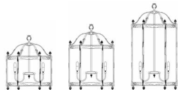
Art. 1881/P ø 63 cm H 76 cm 6 x E27 x 40W
