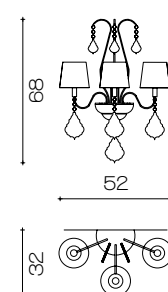
Art. 1742/A3/KR ø 52 cm H 68 cm Pø 14 cm 3 x E14 x 25W
