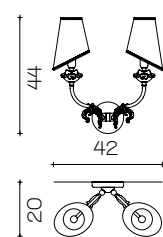
Art. 1774/A2 H 44 cm ø 42 cm Pø 14 cm 2 x E14 x 40W
