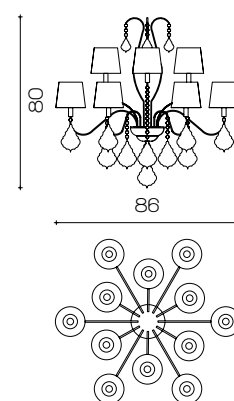
Art. 1742/CH12/KR/V2 ø 86 cm H 80 cm Pø 14 cm 8 x E14 x 25W
