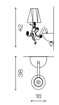
Art. 1631/A1 PØ 16 cm H 42 cm Sp 38 cm 1 x E14 x 40W
