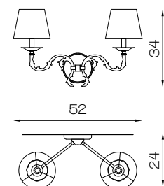
Art. 1986/A2 ø 52 cm H 34 cm Pø 16 cm 2 x E14 x 40W
