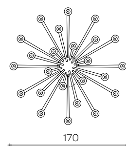
Art. 1761/CH24 Ø 170 cm H 215 cm Pø 16 cm 24 x E14 x 40W
