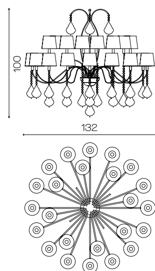
Art. 1742/CH24/KR ø 132 cm H 100 cm Pø 14 cm 24 x E14 x 25W
