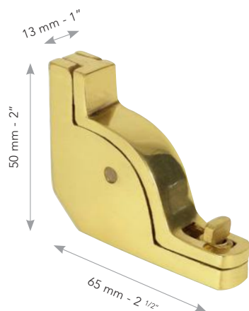
Pour tube For profile x 2 66344
