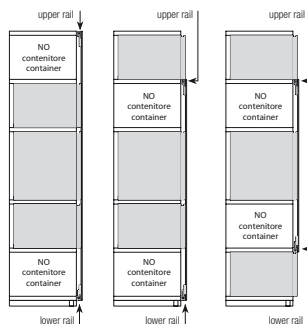
Contenitore avanzato per frontale "CON BATTUTA 3 LATI" Container with external front "WITH REBATE ON 3 SIDES"
