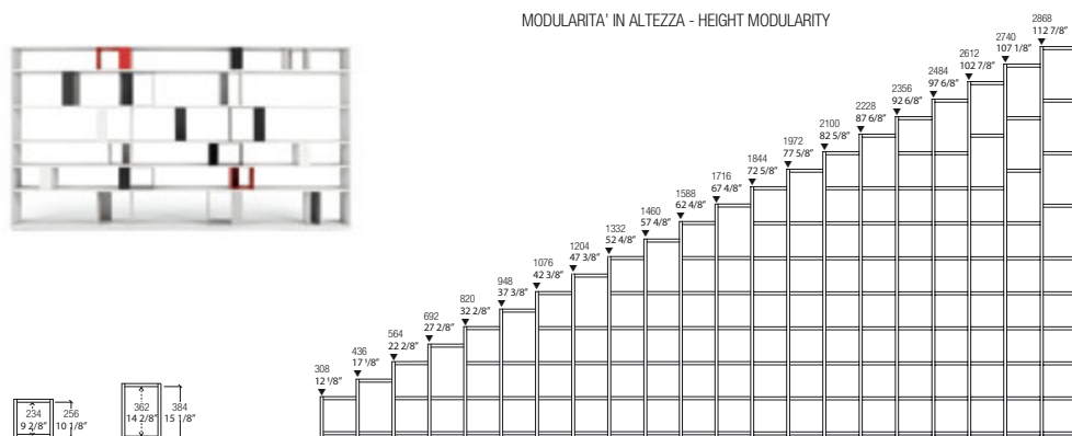
SCHEMA DI UTILIZZO CONTENITORI CON ANTE SCORREVOLI DIAGRAM ON THE USE OF CONTAINERS WITH SLIDING DOORS
