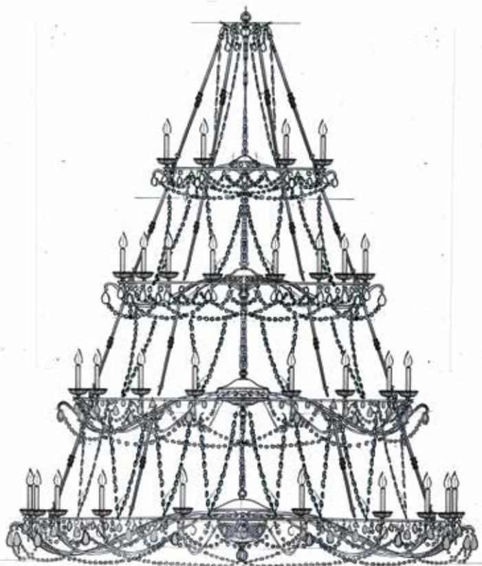
Lampadario 60 luci con strass ottagoni di mm30 e mm25 Gocce di mm64 e 80 Struttura in ferro a foglia oro o argento Bobeche in cristallo molato particolari in fusione di bronzo.
