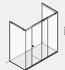
Flat D – F2 Esempio di doccia a tre lati con anta scorrevole example for shower with three sides and sliding door
