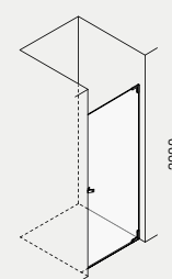
Flat D – B1 Esempio di doccia in nicchia con anta a battente example for shower in niche with hinged door
