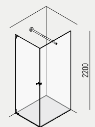
Flat D – C1 Esempio di doccia ad angolo con anta a battente example for corner shower with hinged door
