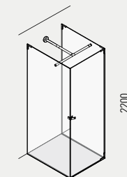
Flat D – D3 Esempio di doccia a tre lati con anta a battente example for shower with three sides and hinged door
