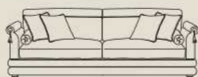
Divano 4 posti 4 Seater-sofa 4-х местный диван L. 260 P. 90 H. 95 NETTO NET NETTO Kg. 90 LORDO GROSS BRUTTO Kg. 96 M 3 2,30
