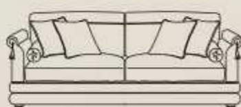
Divano 3 posti 3 Seater-sofa 3-х местный диван L. 220 P. 90 H. 95 NETTO NET NETTO Kg. 62 LORDO GROSS BRUTTO Kg. 62,50 M 3 1,90
