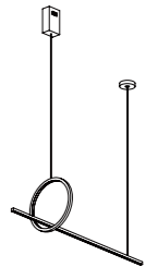
MD1824A-300 3014#25W L1000*W300*H1500
