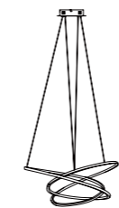
MD1603A-7A 3014#50W L720*W720*H1500
