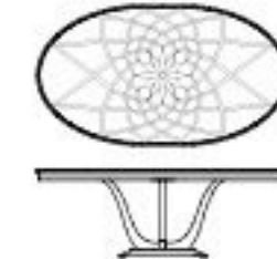
TAVOLO / TABLE P618/V - 225x125x76 h. cm
