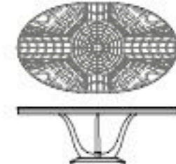
TAVOLO / TABLE P617/V - 225x125x76 h. cm
