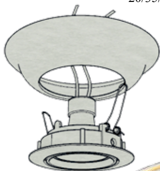
957 - C1 D6 A7 cm d11,5xh3,5 foro-hole-отверстие cm d.6,5 lampadina dicroica - dichroic bulb - встроенный светильник галогенный 20/35/50 watt
