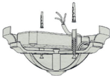
Schema di montaggio Installation diagram Схема монтажа
