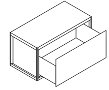
1 drawer (h 21 5/8") w 18", 23 5/8", 29 1/2", 35 1/2", 41 1/4", 47 1/4"
