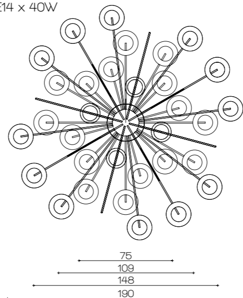
Art. 1451/CH32 ø 190 cm H 185 cm 32 x E14 x 40W
