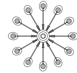
Art. 1774/CH12 ø 110 cm H 66 cm Pø 14 cm 12 x E14 x 40W
