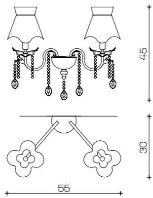
Art. 1689/A2 L 55 cm H 45 cm Sp 30 cm Pø 18 cm 2 x E14 x 40W
