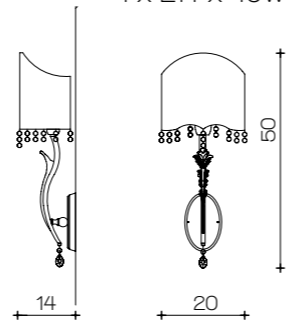
Art. 1689/A1/V2 L20 cm H 50 cm Sp 14 cm 1 x E14 x 40W
