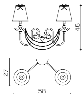
Art. 1794/A2 L 58cm H 45 cm Sp 27 cm Pø 16 cm 2 x E14 x 40W
