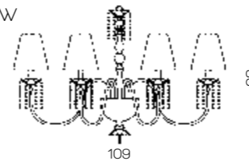
Art. 1506/CH8 ø 109 cm H 68 cm Pø 16 cm 8 x E14 x 40W
