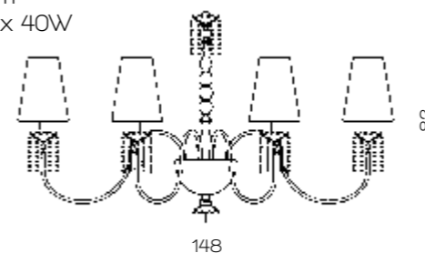
Art. 1507/CH8 ø 148 cm H 82 cm Pø 18 cm 8 x E14 x 40W
