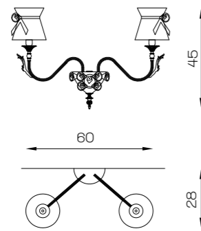
Art. 1850/A2 L 60 cm H 45 cm Sp 28 cm 2 x E14 x 40W
