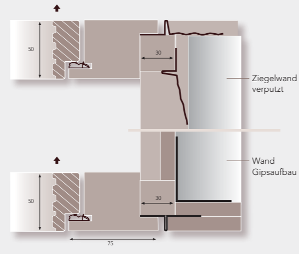
M-Zarge mit Blindstock
