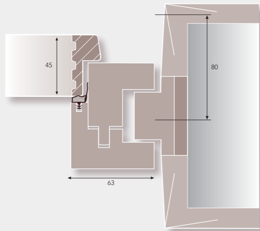
Zweiteiliger Pfostenstock mit Türblatt 45 mm
