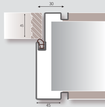
Edelstahlzarge bündig mit Türblatt und Mauer
