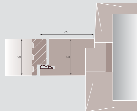
M-Zarge mittig Mauer
