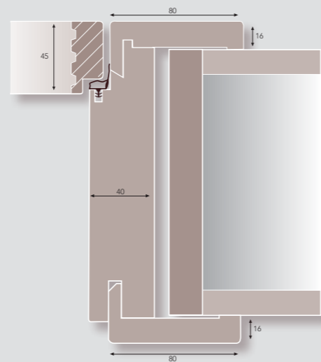
Futterstock 40 mm mit Türblatt 45 mm flächenbündig
