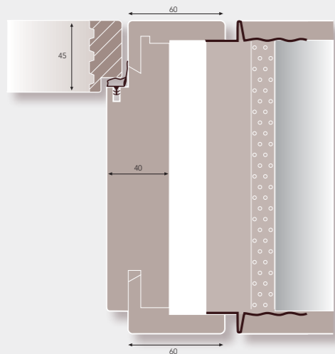
F-Zarge mit Blindstock
