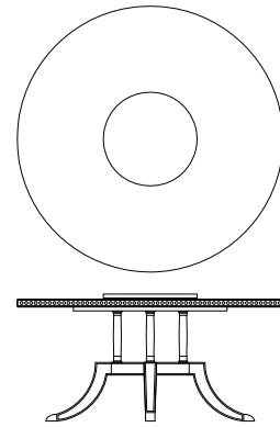
T 900 CAESAR TAVOLO TABLE Ø CM 170XH79 (CM 3 TOP GIREVOLE/ROUND TOP)
