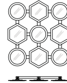
CAESAR COMPOSIZIONE 1 COMPOSITION 1 SPECCHIERA MODULARE GIREVOLE REVOLVING MODULAR MIRROR CM 87XH95
