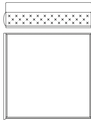
B 650 SARAYA SOMMIER CAPITONNÉ CON RETE ORTOPEDICA A SOLLEVAMENTO PER LETTO CONTENITORE SOMMIER CAPITONNÉ WITH LIFTING ORTHOPAEDIC SPRING FOR BED CONTAINER CM 210X205XH36 MATERASSO MATTRESS CM 200X200
