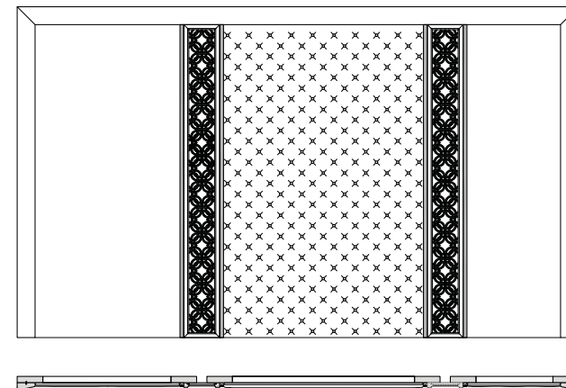
SARAYA TESTATA LETTO COMPONIBILE MODULARHEADBOARD CM 438X10XH258
