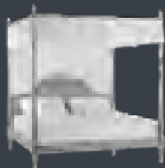
Art. 441/1 Dim. cm 214 x 211 x 240 h Finitura/Finish Tortora/ bianco N° 405
